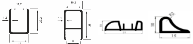
MTCK-020 SÜRGÜLÜ SİSTEM DIŞ YAN PROFİLİ MTCK-021 SÜRGÜLÜ SİSTEM İÇ YAN PROFİLİ MTCK-022 MANYETİK DUVAR DİKME PROFİLİ MTCK-023 ÜÇGEN ALT ÇITA PROFİLİ
